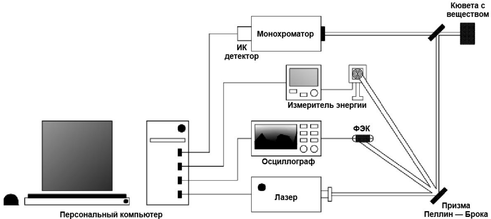
Схема экспериментальной установки
